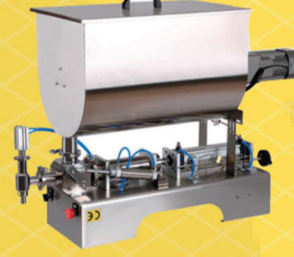
ماكينة تعبئة سوائل بستم-تلك تسخين liquids filling machine biston double jacket tank
