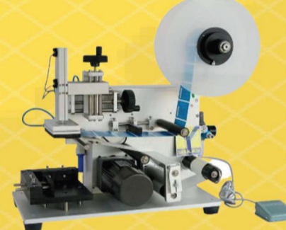
ماكينة ليبل مسطح نص الي Semi-auto square labeling machine
