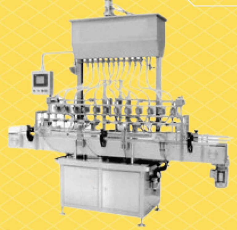
ماكينة تعبئة سوائل خفيفة 10 نزل اتوماتيك Automatic 10 nozzle filling machine
