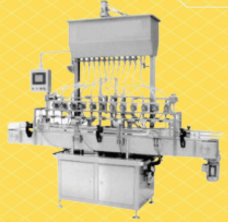
ماكينة تعبئة سوائل خفيفة 10 نزل اتوماتيك Automatic 10 nozzle filling machine
